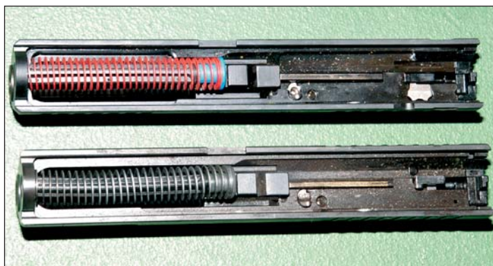
Zoek de verschillen tussen de Q-NL slede (boven) en die van een civiele P99 AS- uitvoering.
